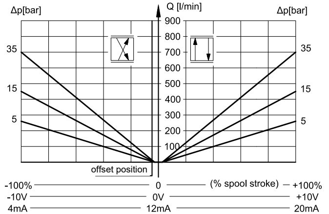
Z250
