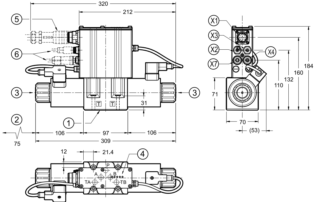
DSE5GH-*/SA/K16
