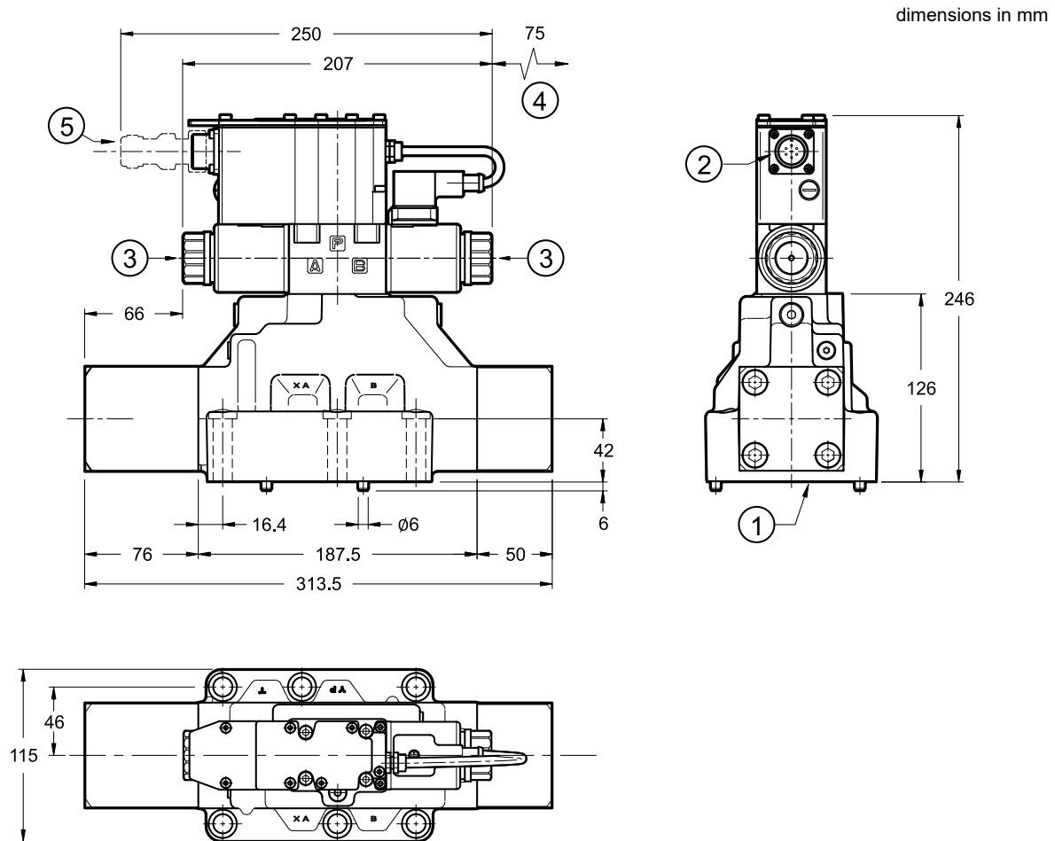
DSPE8GL
