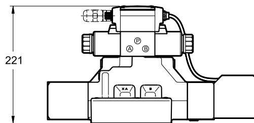
DSPE8JL
