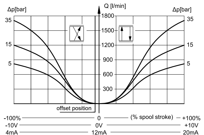
Z800
