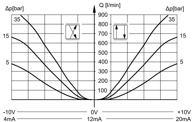
C400 / A400
