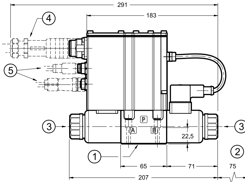
ZDE3GH-D/*K16
