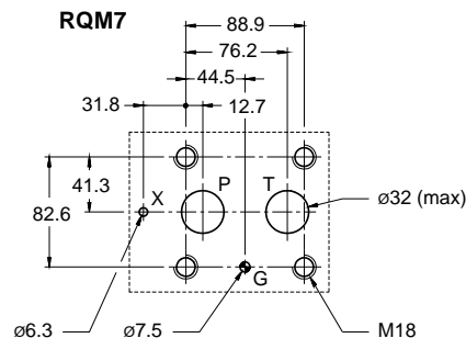
RQM7
