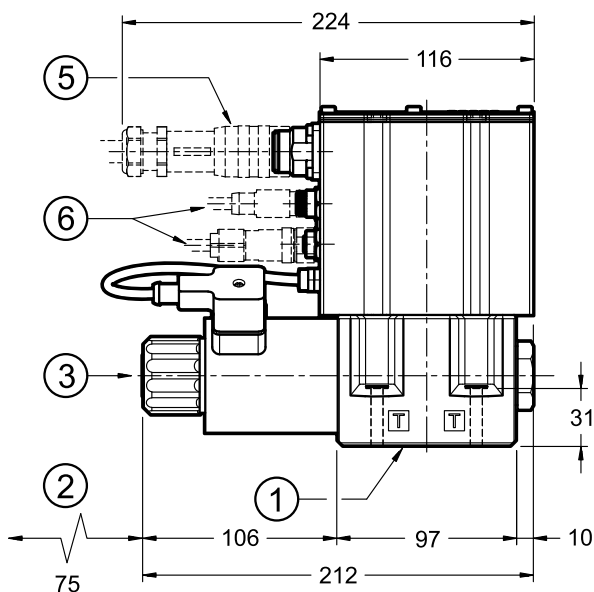
DSE5GH-*/SA/K16
