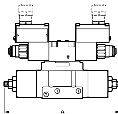
DSP*K*-/C
