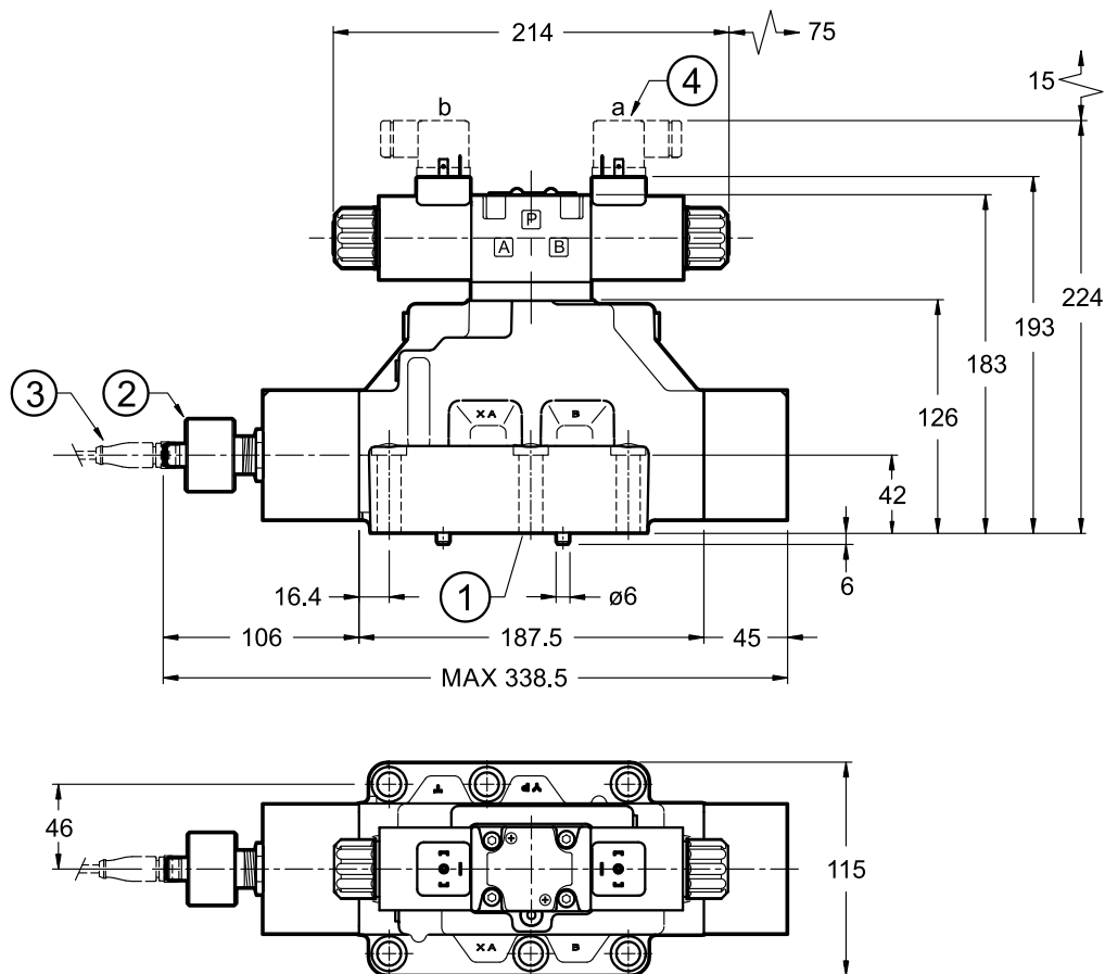
DSP8M-RK
