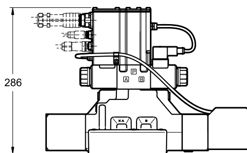
DSPE8JH
