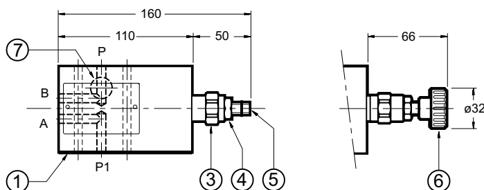
RPC1-K/M/PCT3
