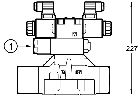
DSPE7
