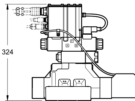
DDPE8JH
