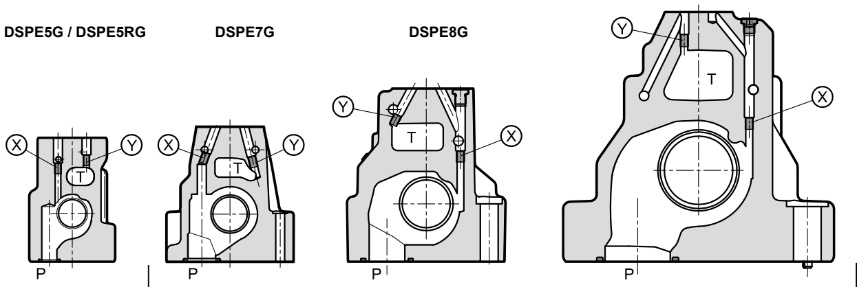
DSPE10/11G
