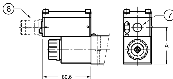
PDE3K* -*K9S*
