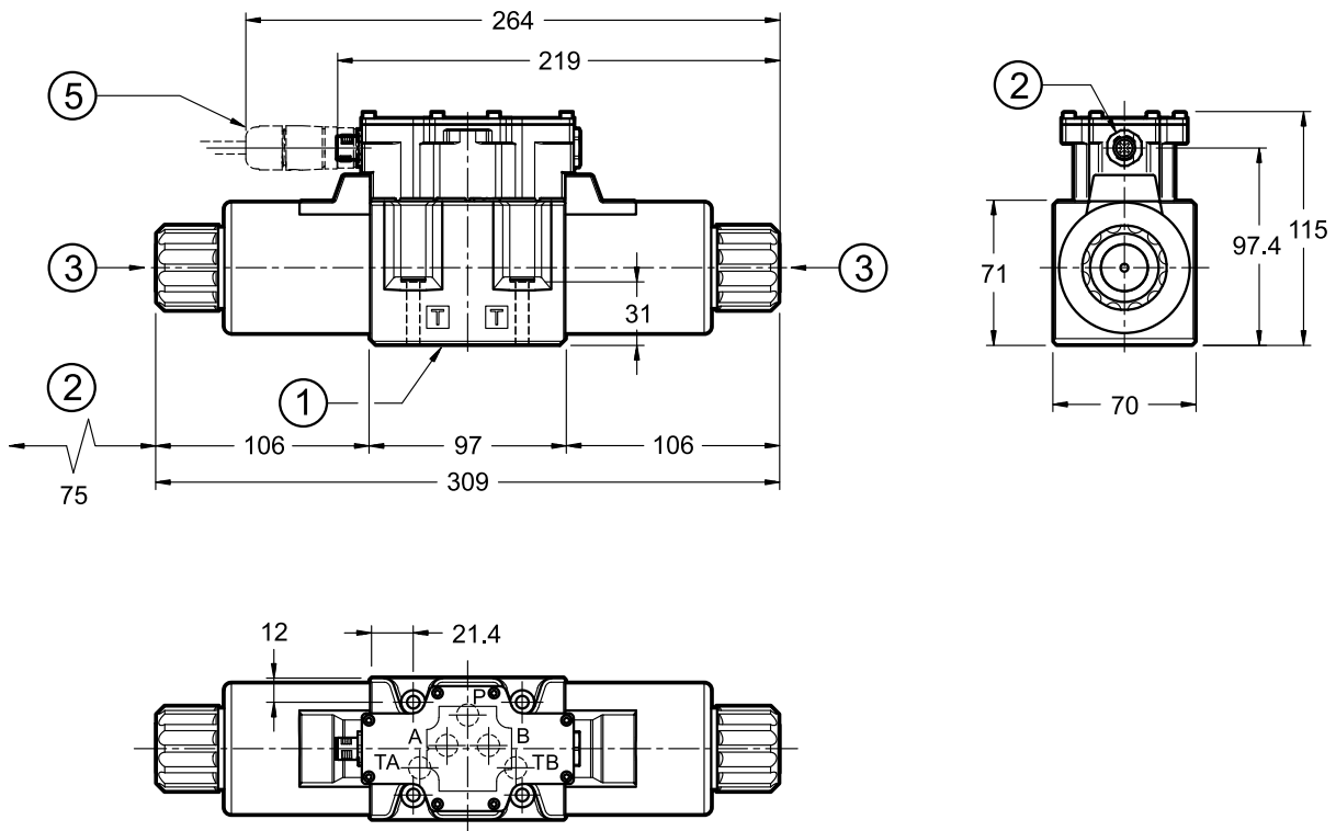
DSE5GL-*/SA/K12
